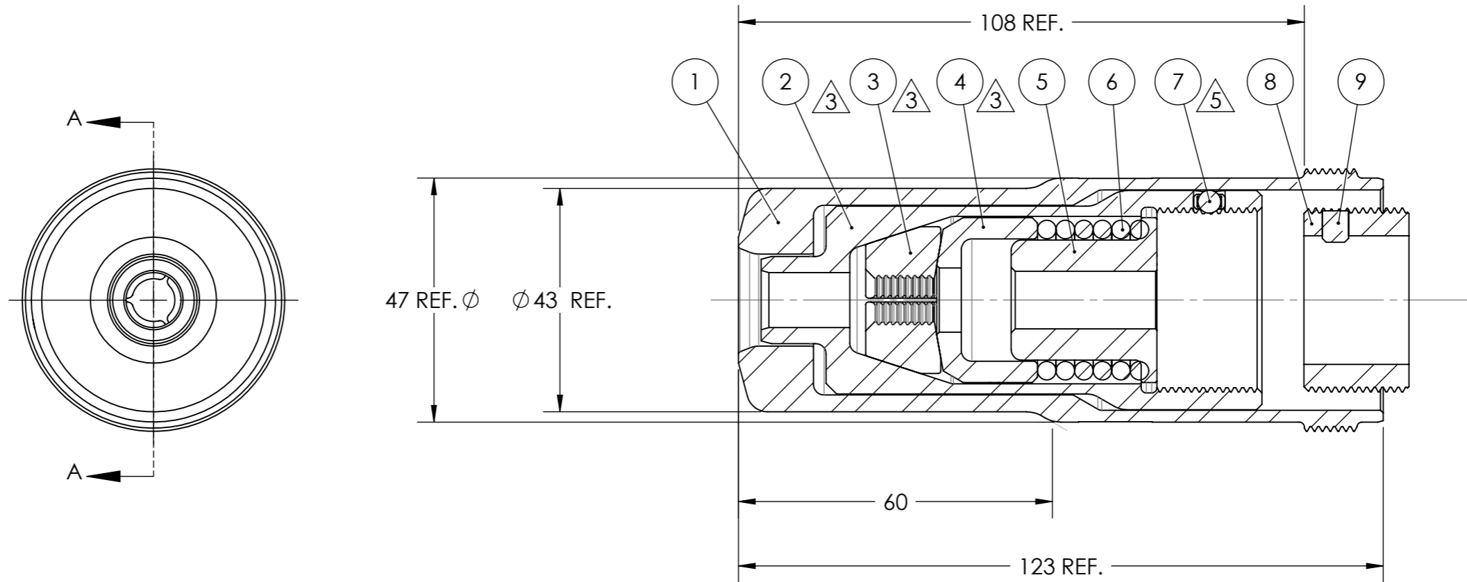
SECTION A-A
